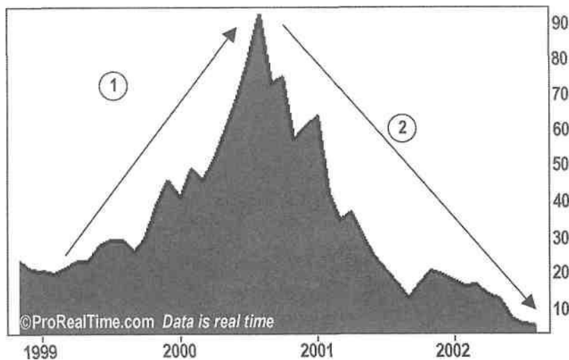
Graphique 8 : Action ALCATEL
